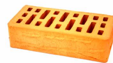
Кирпич одинарный лицевой пустотелый (крупный рельеф)
